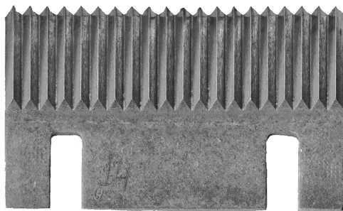
Р и с. 1. Внешний вид свеклорезального ножа F i g. 1. Original appearance of a beet-cutter knife
