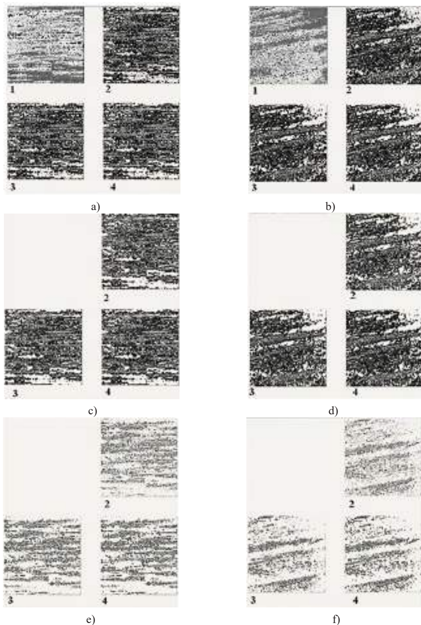
Р и с. 5. Распределения расчетных абсолютных значений показателей, характеризующих процесс трения на поверхности металла ножей без упрочнения (а, с, е) и после упрочнения (b, d, f):
