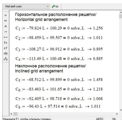
Р и с. 5. Определение минимально допустимой длины перфорированной решетки в программе Mathcad F i g. 5. Determination of the minimum allowable length of a perforated grid in the Mathcad program
