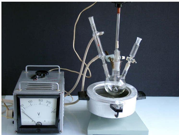
Р и с. 1. Лабораторная установка для получения стабилизатора F i g. 1. Laboratory installation for stabilizer production
