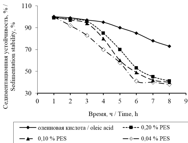
Р и с. 2. Стабилизационные свойства полиэтиленгликольсебацината в сравнении с олеиновой кислотой при разном количестве (мас. %) стабилизатора
